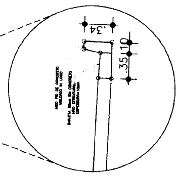
03 - DETALHE MEIO FIO ESC. 5/ESC.
