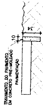
01 - DETALHE MEIO FIO ESC. 5/85C
