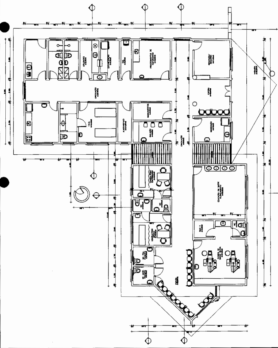
01 PLANTA BAIXA - LAYOUT ÁREA TOTAL CONSTRUIDA = 319,65MP ESCALA = 1/100
