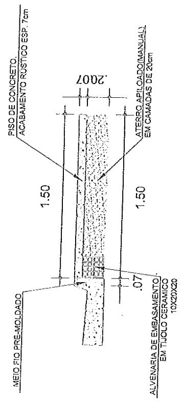
DETALHE CALÇADA Escala = 1/25
