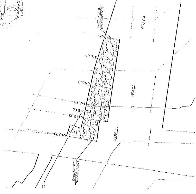
PLANTA BAIXA GEORREFERENCIADA Escala = 1:1000
