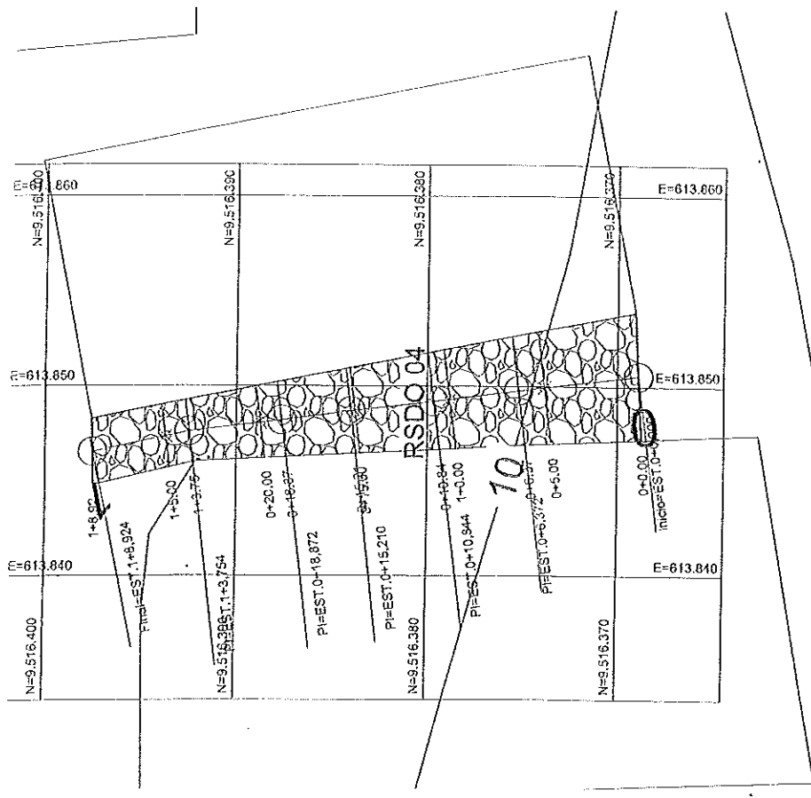
PLANTA BAIXA GEORREFERENCIADA Escala = 1:250
