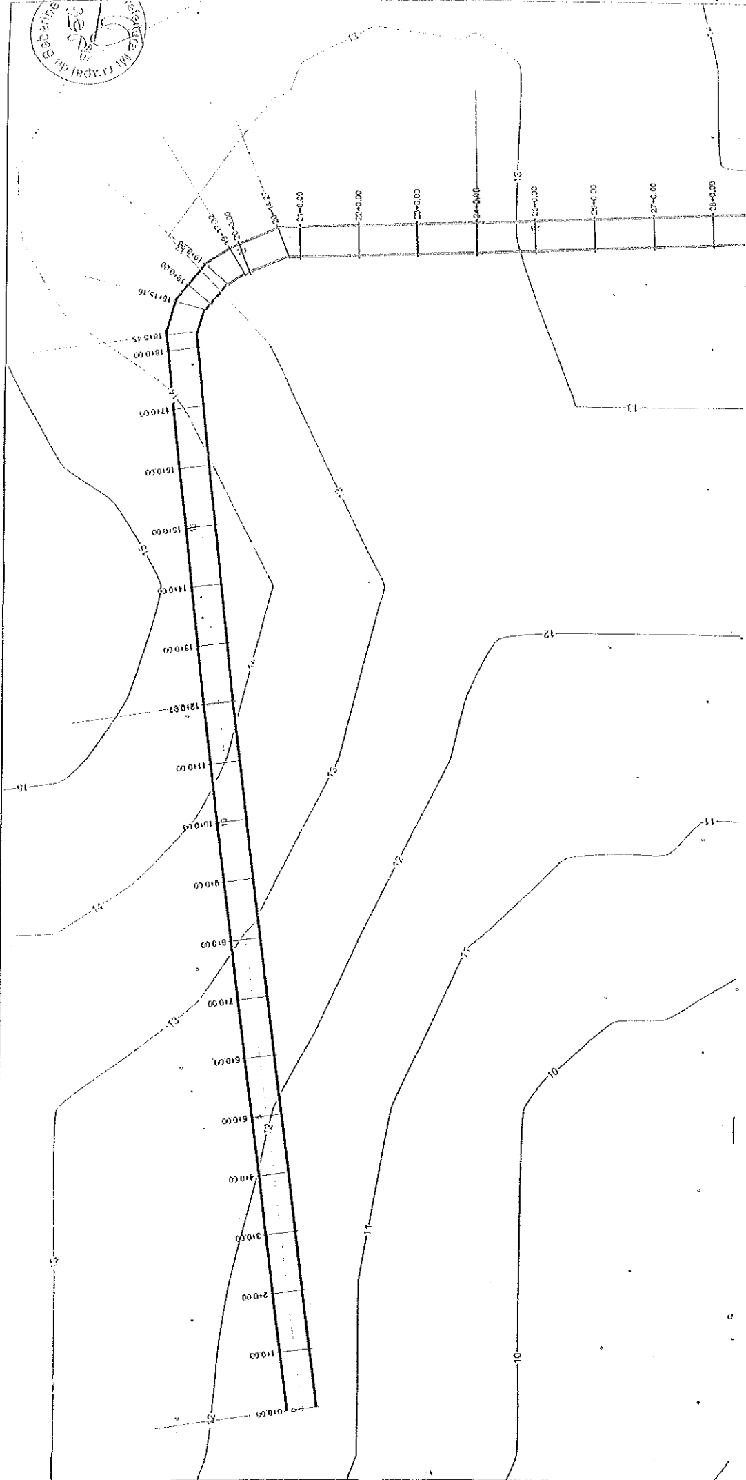
PLANTA BAIXA - TRAÇADO DAS SEÇÕES TRANSVERSAIS Escala = 1:1250
