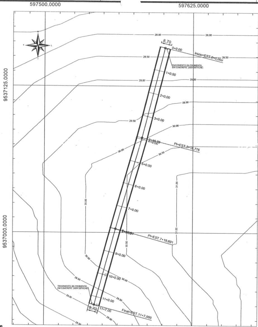
01 - PLANTA PLANIALTIMETRICA GEORREFERENCIADA ESC.: 1/1250
