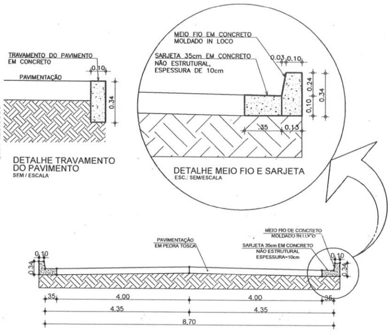
02 - SEÇÃO TIPO ESC.: 1/75
