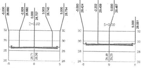
02 - SEÇÕES TRANSVERSAIS ESC.: 1/300
