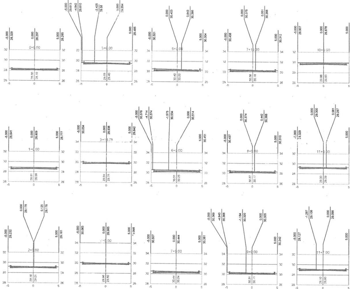
01 - SEÇÕES TRANSVERSAIS ESC.: 1/300
