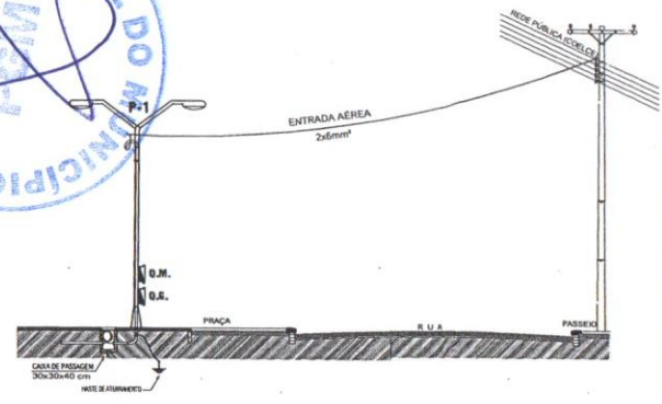
02 DETALHE DA ENTRADA ENERGIA Escala - SEM
