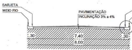
02 - VISTA DE SEÇÃO PADRÃO ESC.: 1/100
