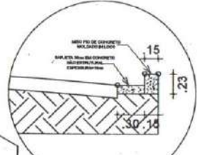
DETALHE MEIO FIO E SARJETA ESCALA: 1/40
