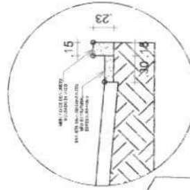
DETALHE MEIO FIO E SARJETETA
