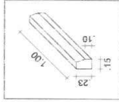
DETALHE MEIO - FIO
