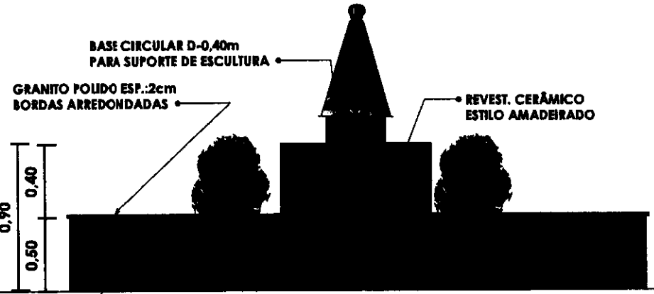
02 VISTA FRONTAL BANCO 03 Escala 1:50
