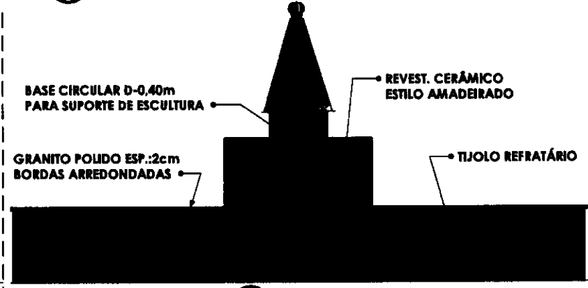
03 VISTA FUNDO BANCO 03 Escala 1:50
