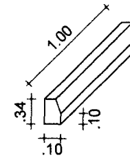
03 - DETALHE MEIO FIO ESC.: 8/ESC.
