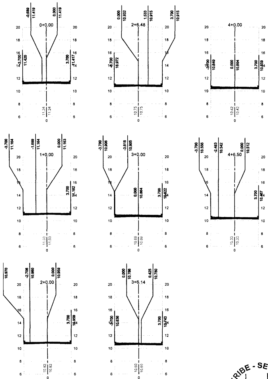
01 - SEÇÕES TRANSVERSAIS Esc.: 1/250
