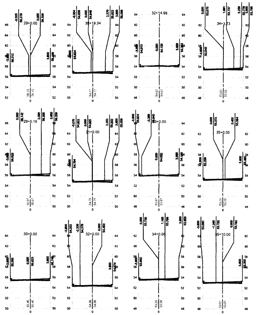
01 - SEÇÕES TRANSVERSAIS - 3ª PARTE Esc.: 1/300
