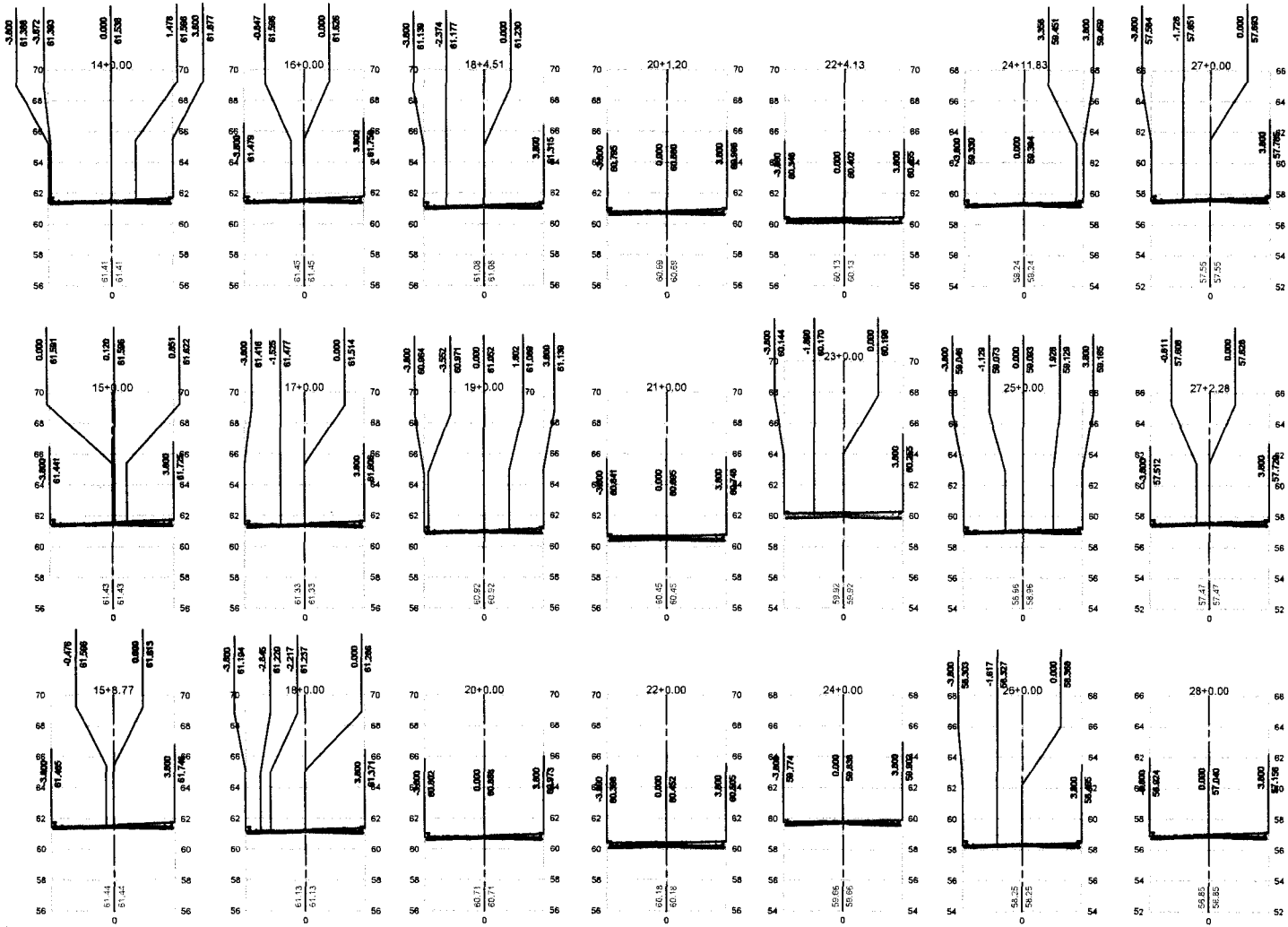
01 - SEÇÕES TRANSVERSAIS - 2a PARTE ESC.: 1/300
