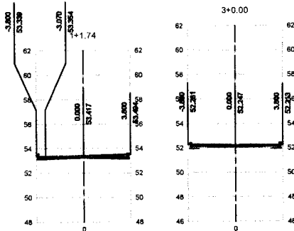
01 - SEÇÕES TRANSVERSAIS - 1ª PARTE ESC.: 1/300
