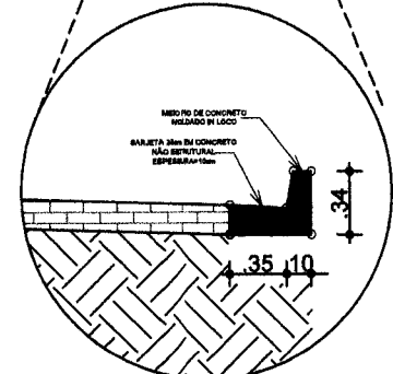
04 - DETALHE MEIO FIO E SARJETA ESC.: 5/ESC.
