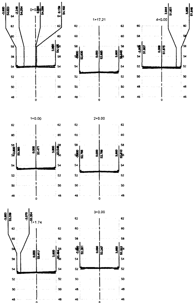
01 - SEÇÕES TRANSVERSAIS - 1a PARTE ESC.: 1/300
