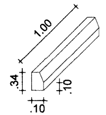
03 - DETALHE MEIO FIO ESC.: 8/ESC.
