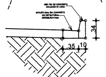
03 - DETALHE MEIO FIO E SARJETA ESC.: 5/ESC.
