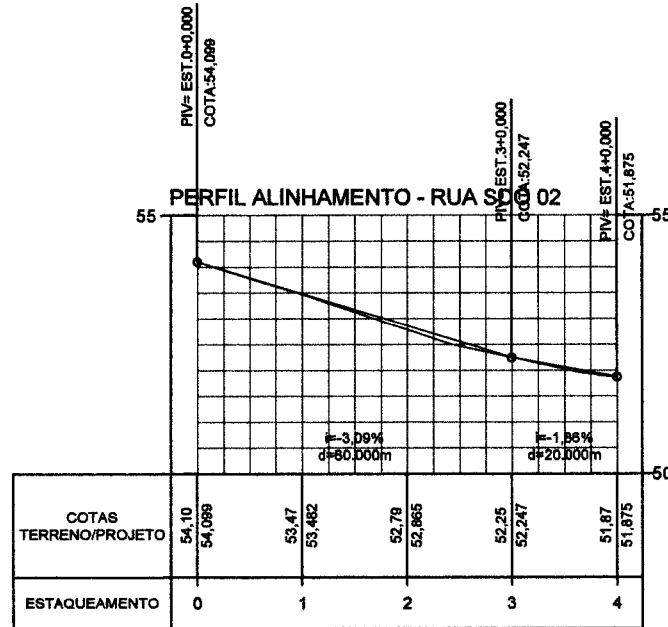
02 - PERFIL LONGITUDINAL ESC.: HORIZONTAL=1/1000 / VERTICAL=1/100
