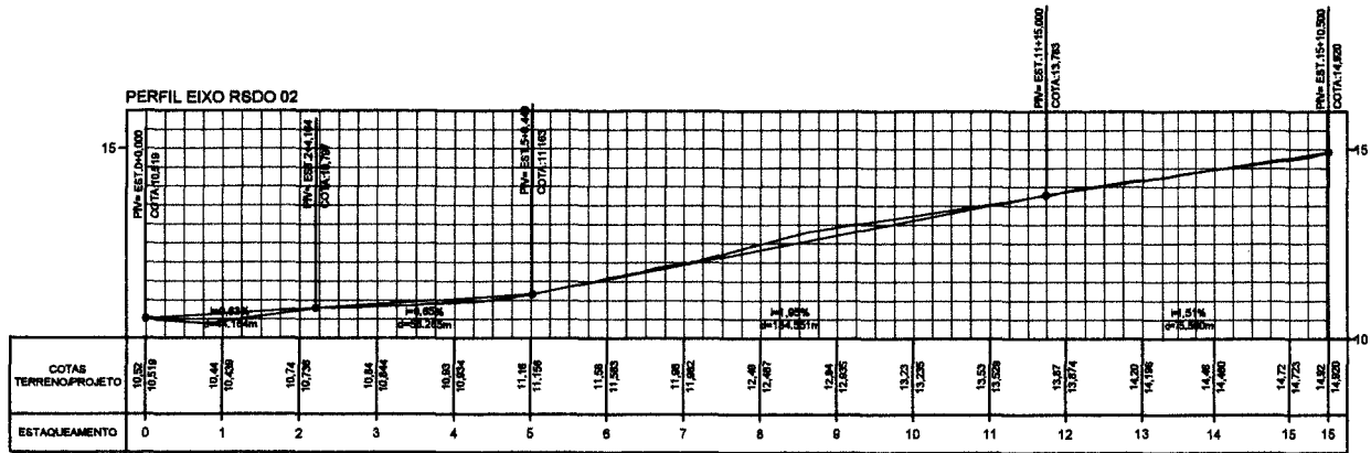
02 - PERFIL LONGITUDINAL ESC.: HORIZONTAL=1/500 / VERTICAL=1/50
