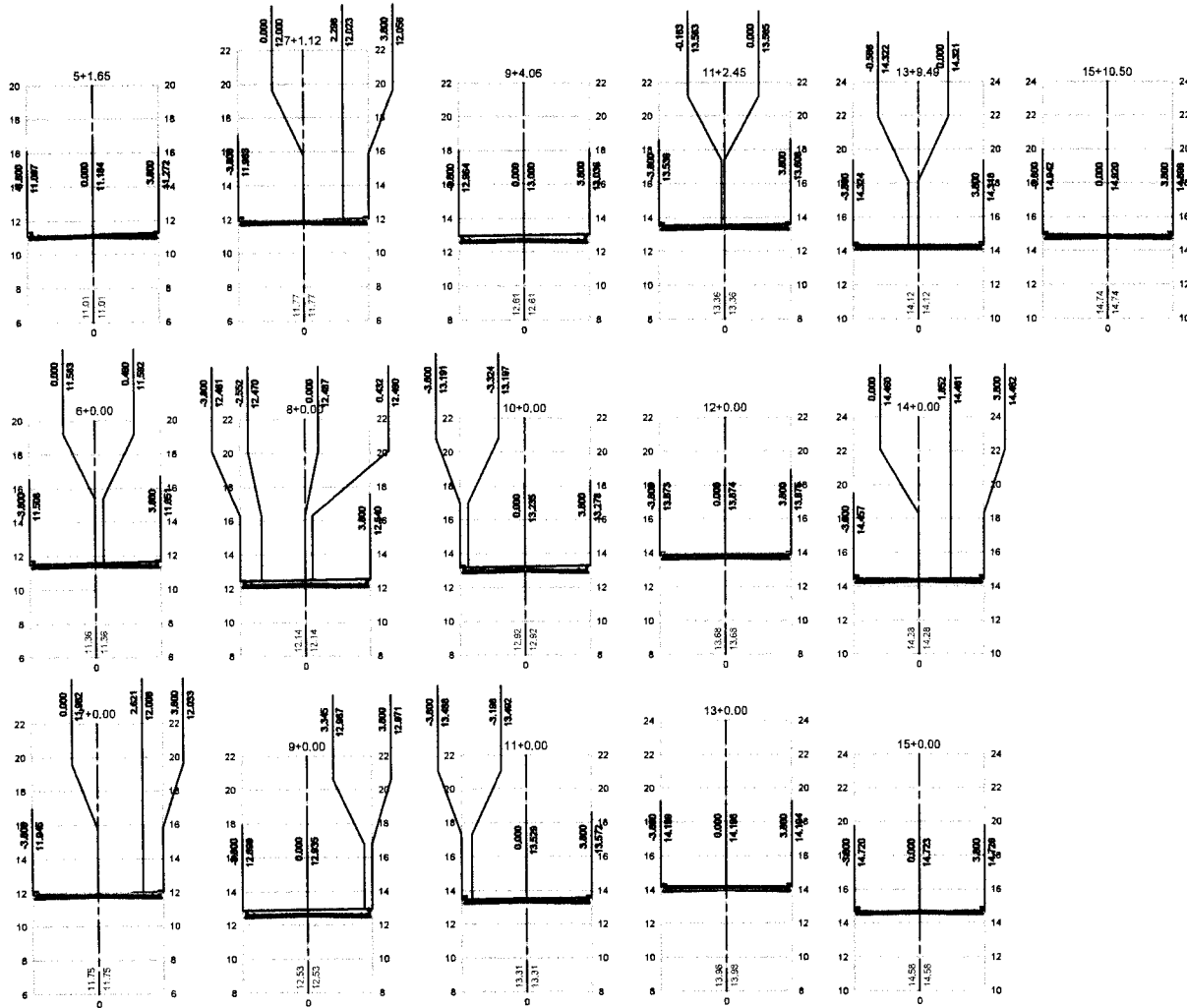
01 - SEÇÕES TRANSVERSAIS - 2a PARTE ESC: 1/300
