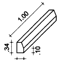
04 - DETALHE MEIO FIO ESC.: 5/ESC.
