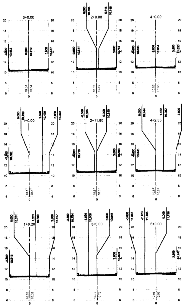
01 - SEÇÕES TRANSVERSAIS - 1ª PARTE ESC.: 1/300
