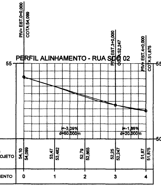
02 - PERFIL LONGITUDINAL ESC.: HORIZONTAL=1/1000 / VERTICAL=1/100
