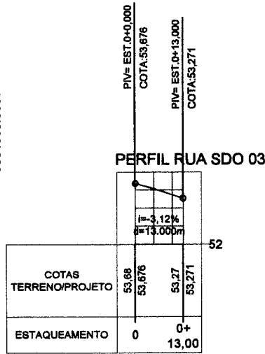
02 - PERFIL LONGITUDINAL ESC.: HORIZONTAL=1/1500 / VERTICAL=1/150
