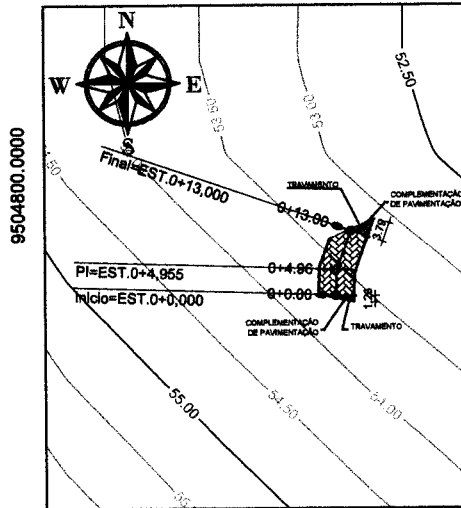
01 - PLANTA PLANIALTIMETRICA GEORREFERENCIADA ESC.: 1/1000
