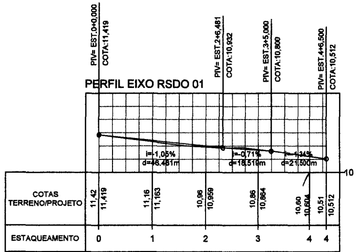
02 - PERFIL LONGITUDINAL ESC.: HORIZONTAL=1/1000 / VERTICAL=1/100
