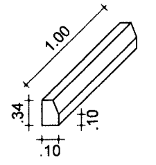
03 - DETALHE MEIO FIO ESC.: 5/ESC.
