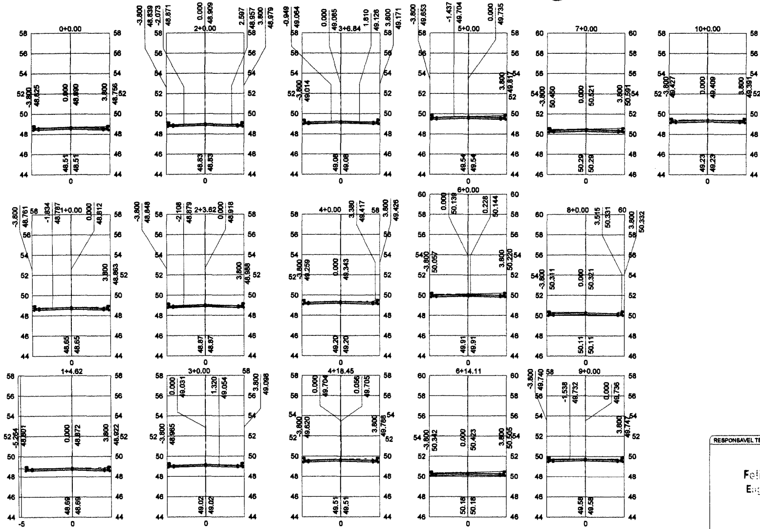
01 - SEÇÕES TRANSVERSAIS ESC.: 1/250
